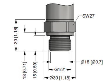
G1/2" DIN 3852 flush p_N \geq 1 \text{ bar}
