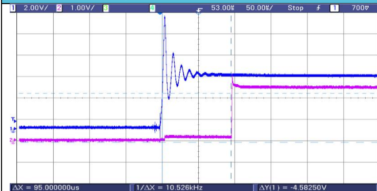
图 7：上电启动 POR 时间图
