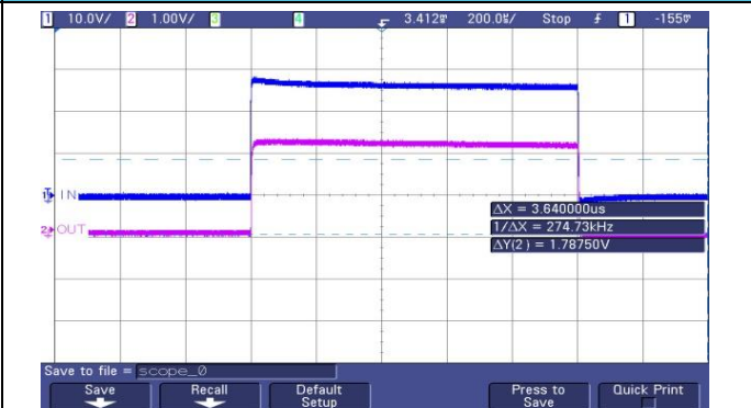
图 6：脉冲瞬态响应图
