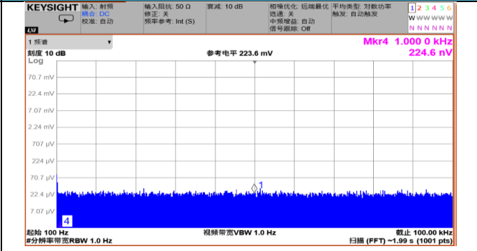
图 4：噪声频谱图
